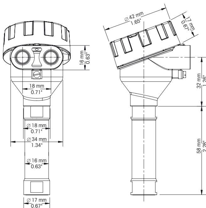
Abmessungen Frontansicht M100
