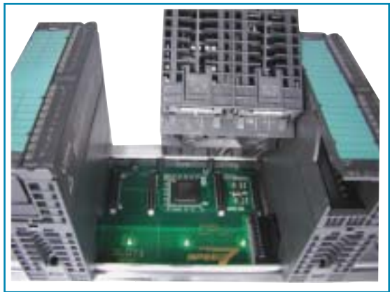
Abbildung Links: Highspeed-Baugruppe auf dem SPEED-Bus von VIPA Mitte: SPEED7-CPU Rechts: Standard-Bus Baugruppe von VIPA oder Siemens
