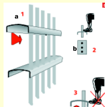
8. a. Außermittige Rundstäbe und Unterbringung des Detektionskabels b. Kaum Trittfläche, das Übersteigen wird stark erschwert
