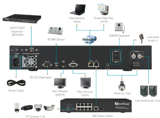
Ansicht Rückseite
