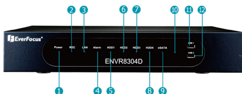
Frontansicht
