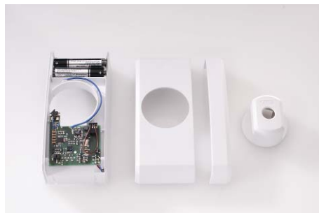
Bereits vorhandene, rein mechanische Fenstersicherungen können schnell zur Funk-Fenstersicherung aufgerüstet werden.
